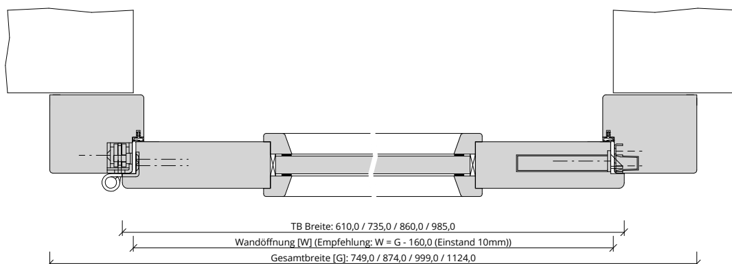
Q_FS_TB-BLE-1FLG_OLMKMQ_GEF_FS-30-1-LA.pdf
