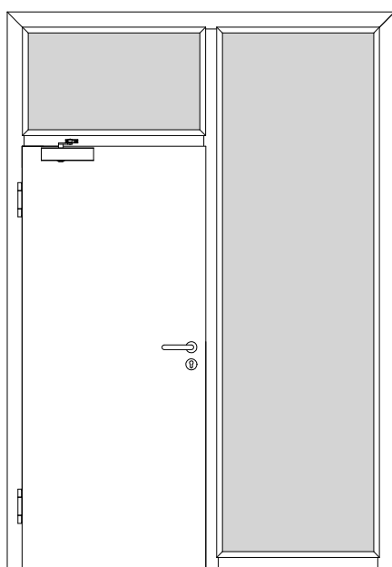
A_FS_TB-BLE-1FLG_WF3-V1_GEF_FS-30-1-RD.pdf
