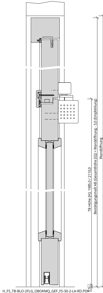
H_FS_TB-BLO-2FLG_OBOKMQ_GEF_FS-30-2-LA-RD.PDF
