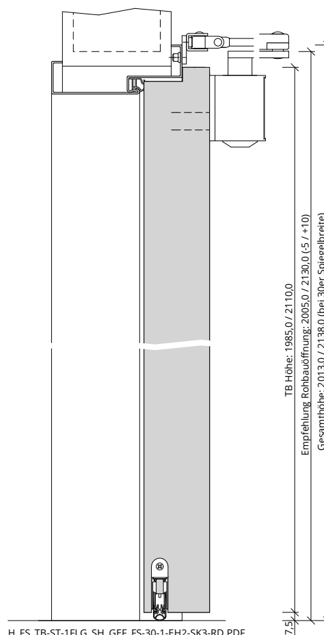
H_FS_TB-ST-1FLG_SH_GEF_FS-30-1-EH2-SK3-RD.PDF
