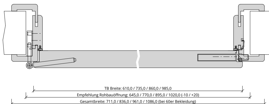
Q_RD_TB-FU-1FLG_SH_GEF_RD-40-HSD.PDF
