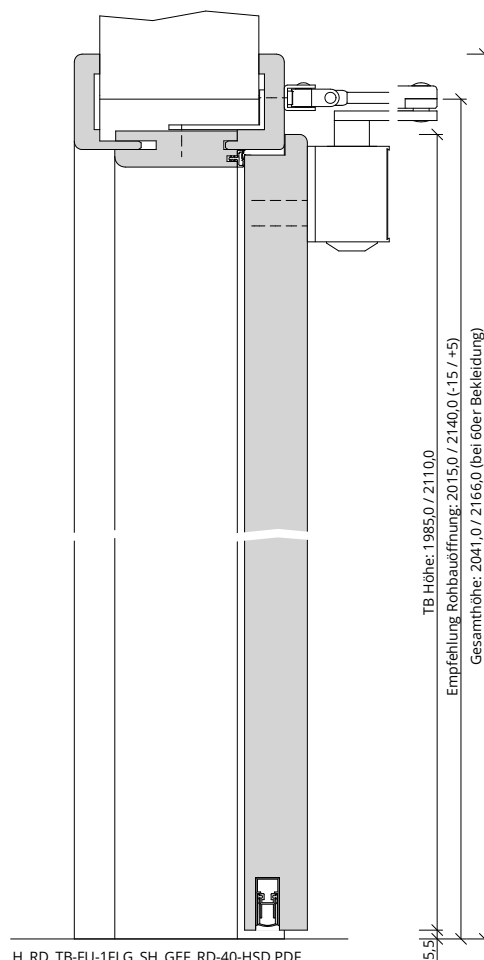
H_RD_TB-FU-1FLG_SH_GEF_RD-40-HSD.PDF
