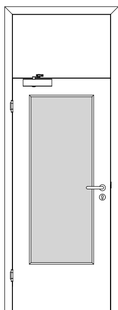
A_RD_TB-BLE-1FLG_OBOKMQ_STU_RD-40-LA.PDF
