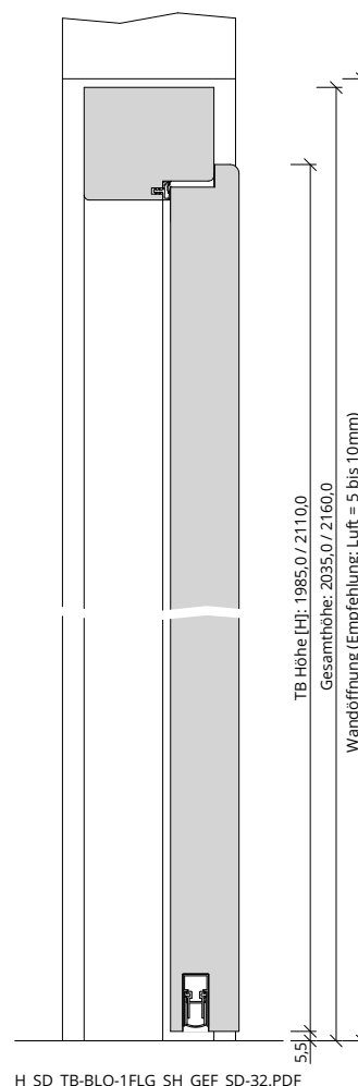
H_SD_TB-BLO-1FLG_SH_GEF_SD-32.PDF
