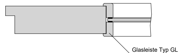
Detail Verglasung
