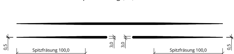
Ansicht Blackline - Spitzfräsung (SF)
