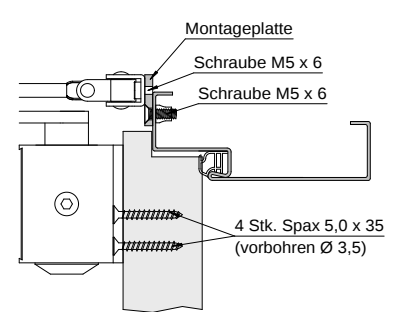
Beispiel Stahlzarge
