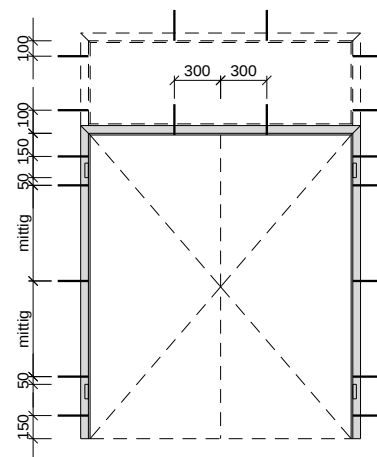
2-flügelig
