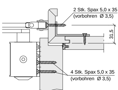
Beispiel Türfutter
