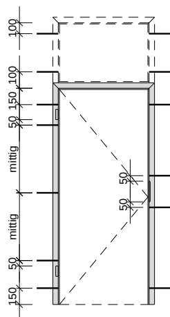
1-flügelig
